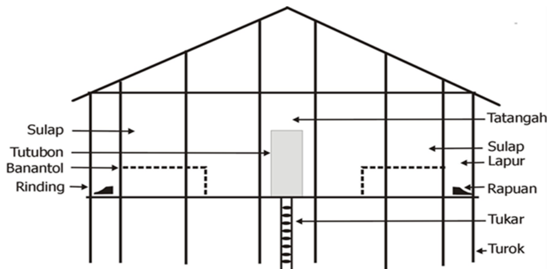
Rajah 1: Pelan Sisi Rumah Panjang Murut Tahol (Mohad Abd Hakim, 2012).
