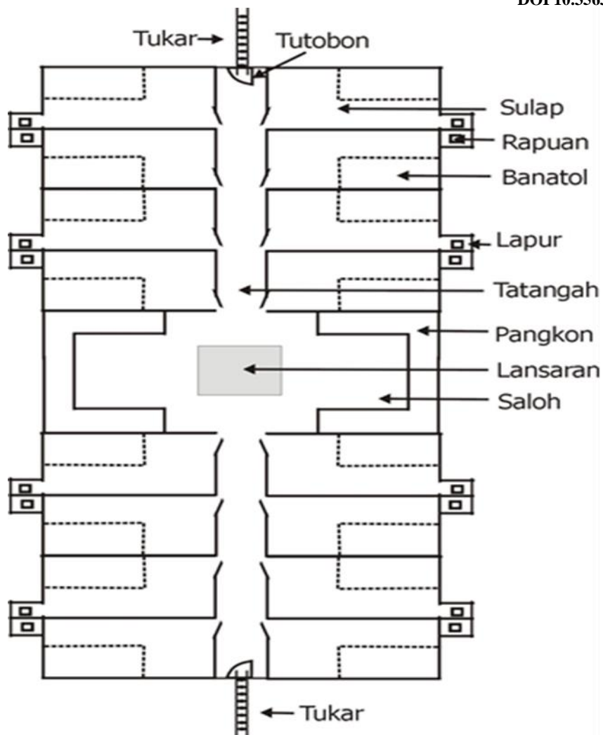
Rajah 2: Pelan Lantai Rumah Panjang Murut Tahol (Mohad Abd Hakim, 2012).
